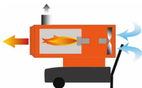
Funktionsweise KS-Serie
